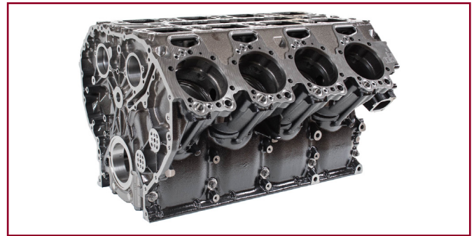
斯堪尼亚(Scania)16升气缸体
