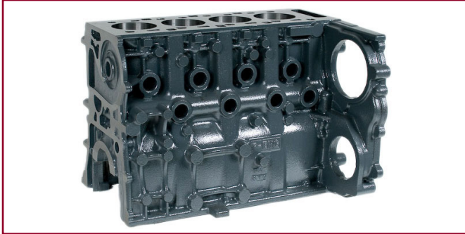
现代3.9升, 5.9升和6.3升气缸体
