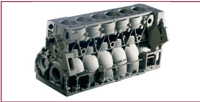
曼(MAN)10.5升和12.4升气缸体 D20和D26发动机
