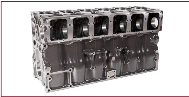
斯堪尼亚(Scania)13升气缸体
