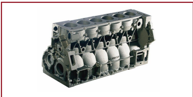
曼 (MAN) 10.5 升和 12.4 升气缸体
